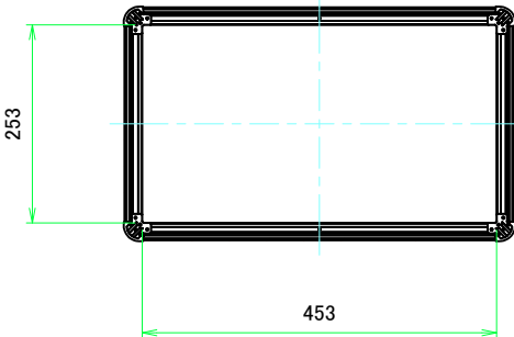
C-C ( 1 : 7.5 )
