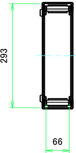
A-A ( 1 : 7.5 )
